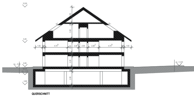
QUERSCHNITT
