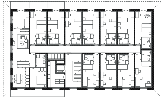
HAUPTHAUS GRUNDRISS OBERGESCHOSS VARIANTE C
